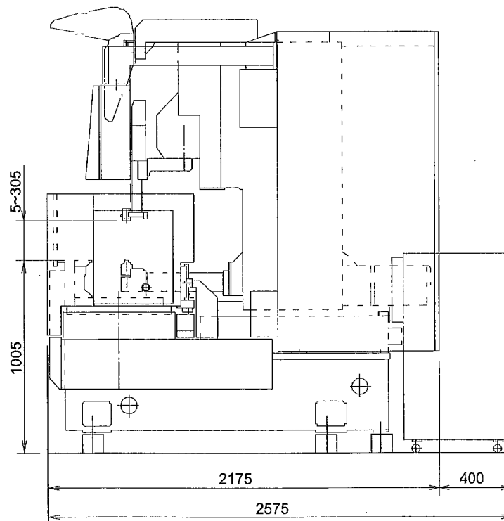
図 2-9 AQ535L 標準タイプ 右側面図
