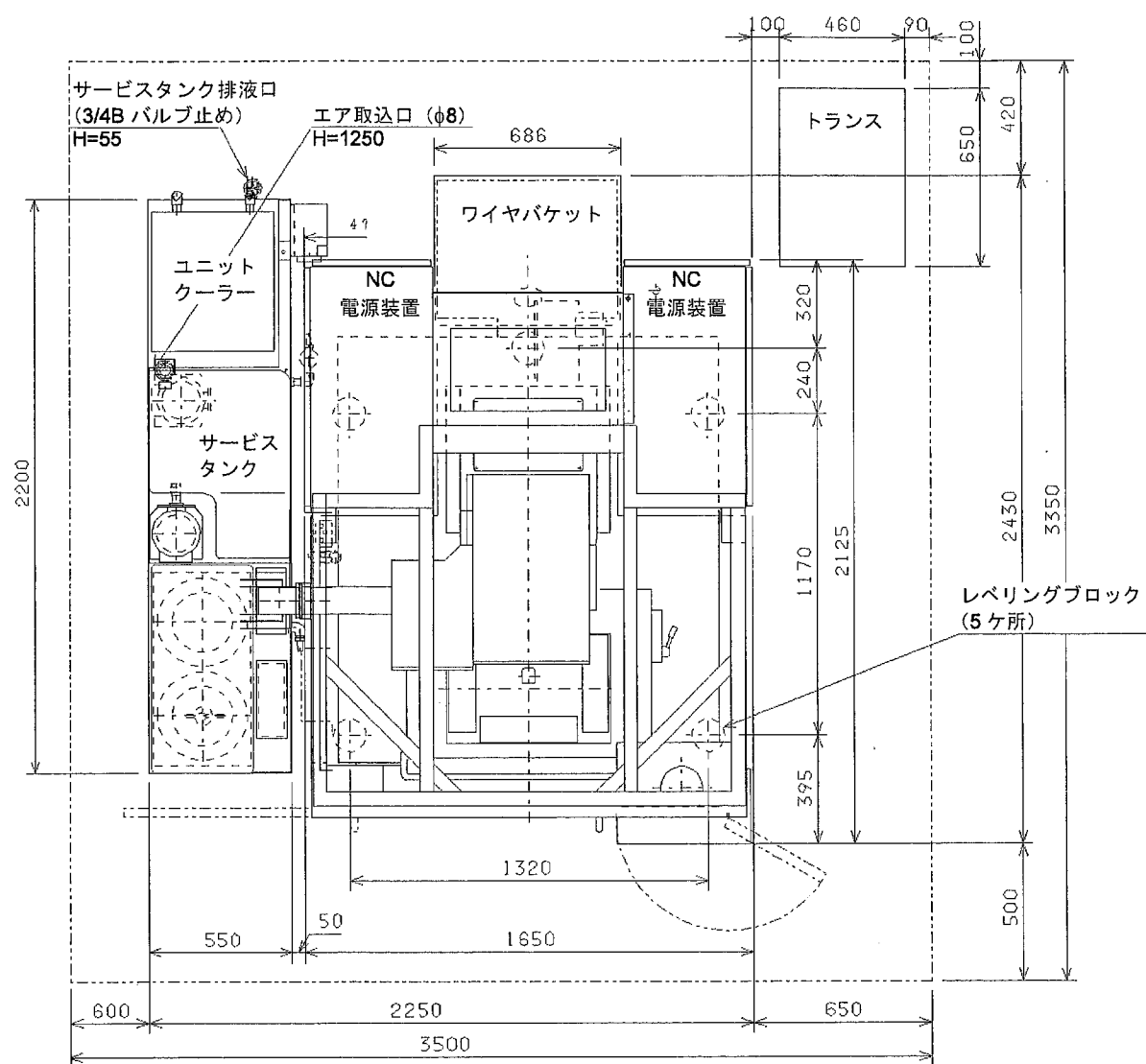
図 2-7 図 AQ325L CE タイプ 配置図
