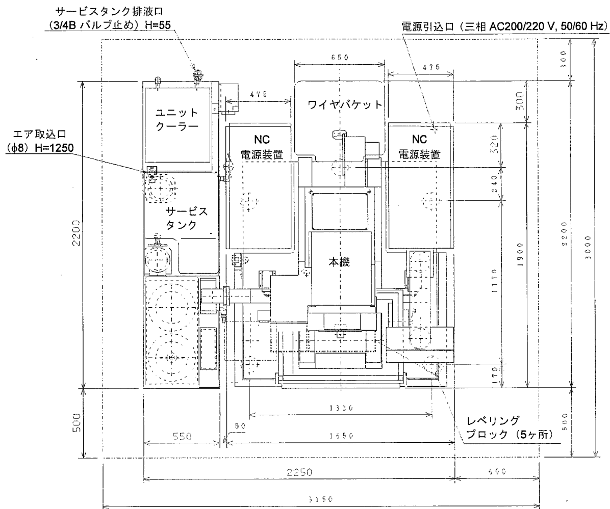
図 2-3 AQ325L 標準タイプ 配置図
