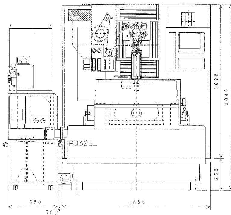
図 2-1 AQ325L 標準タイプ 正面図
