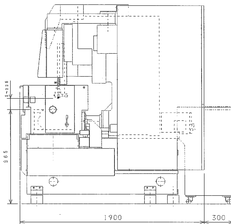
図 2-2 AQ325L 標準タイプ 右側面図
