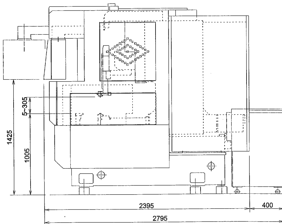
図 2-13 AQ535L CE タイプ 右側面図
