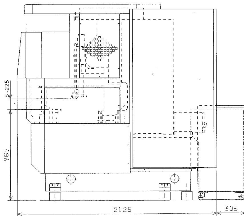
図 2-6 AQ325L CE タイプ 右側面図
