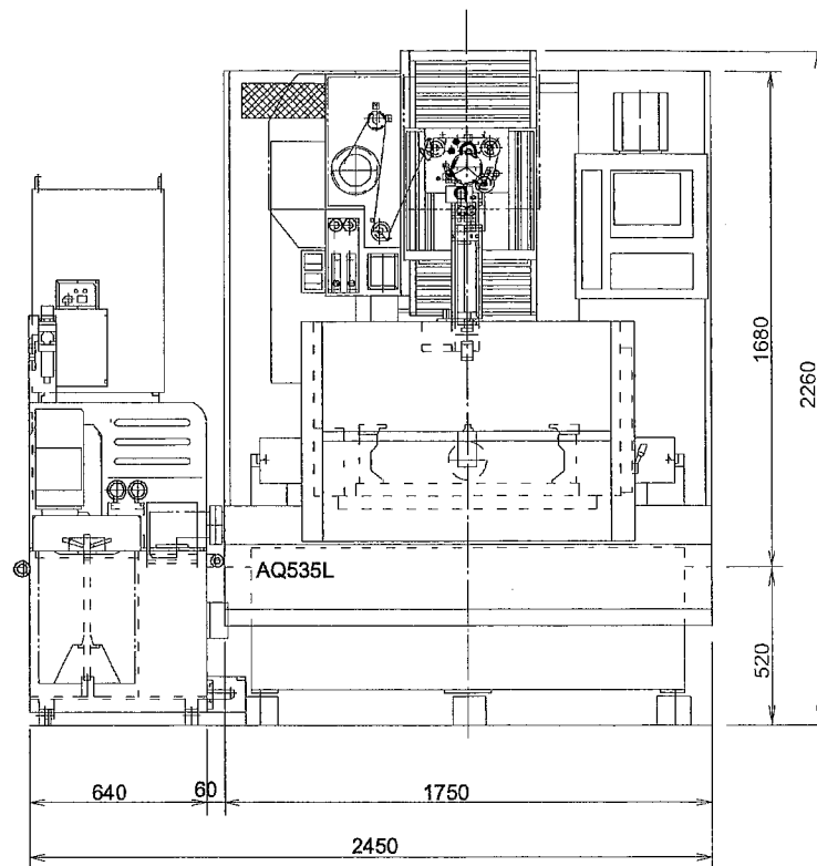
図 2-8 AQ535L 標準タイプ 正面図
