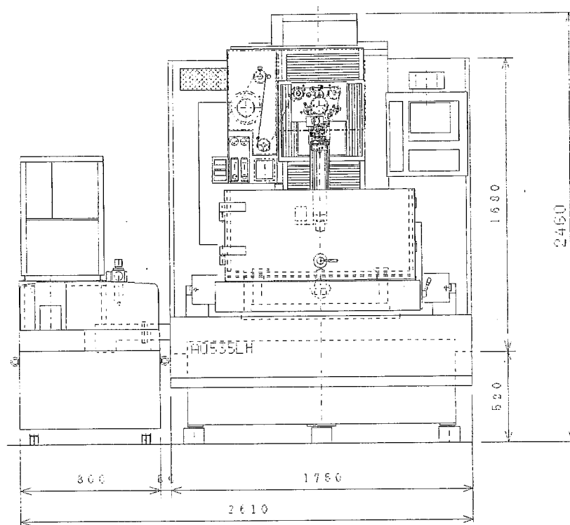
図 2-15 AQ535LH 正面図
