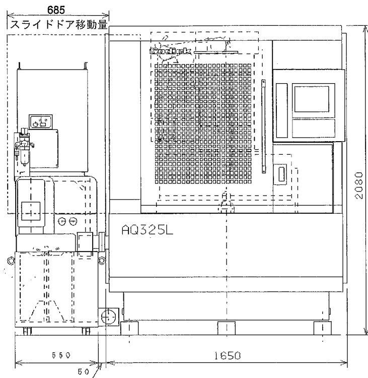
図 2-5 AQ325L CE タイプ 正面図
