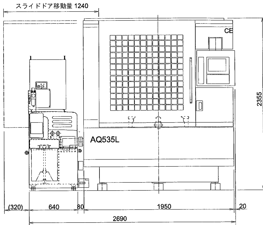
図 2-12 AQ535L CE タイプ 正面図
