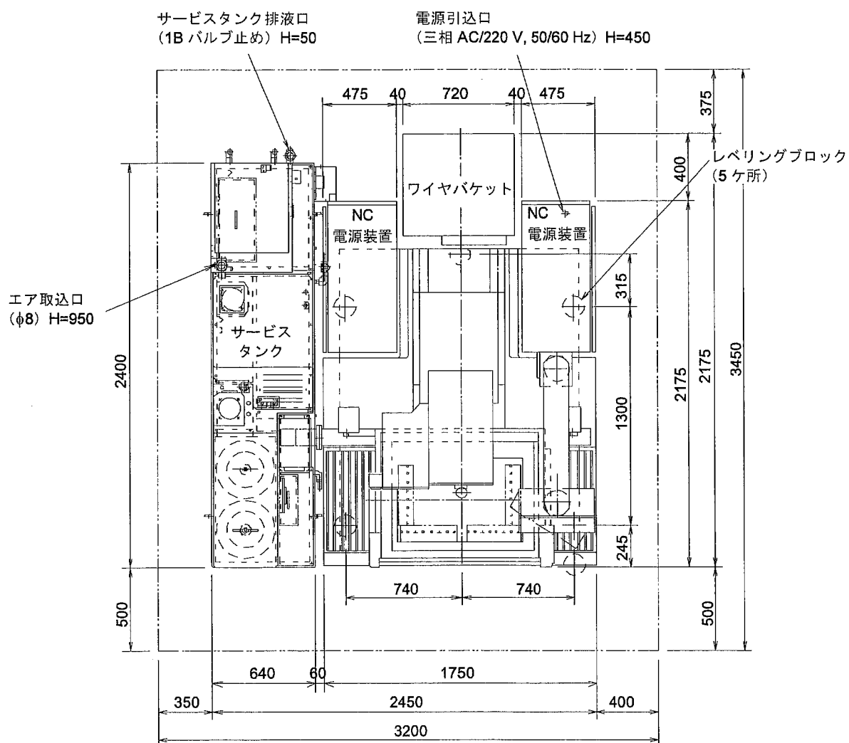
図 2-10 AQ535L 標準タイプ 配置図
