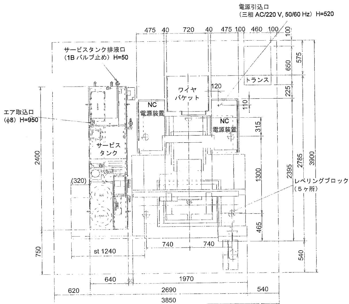
図 2-14 AQ535L CE タイプ 配置図
